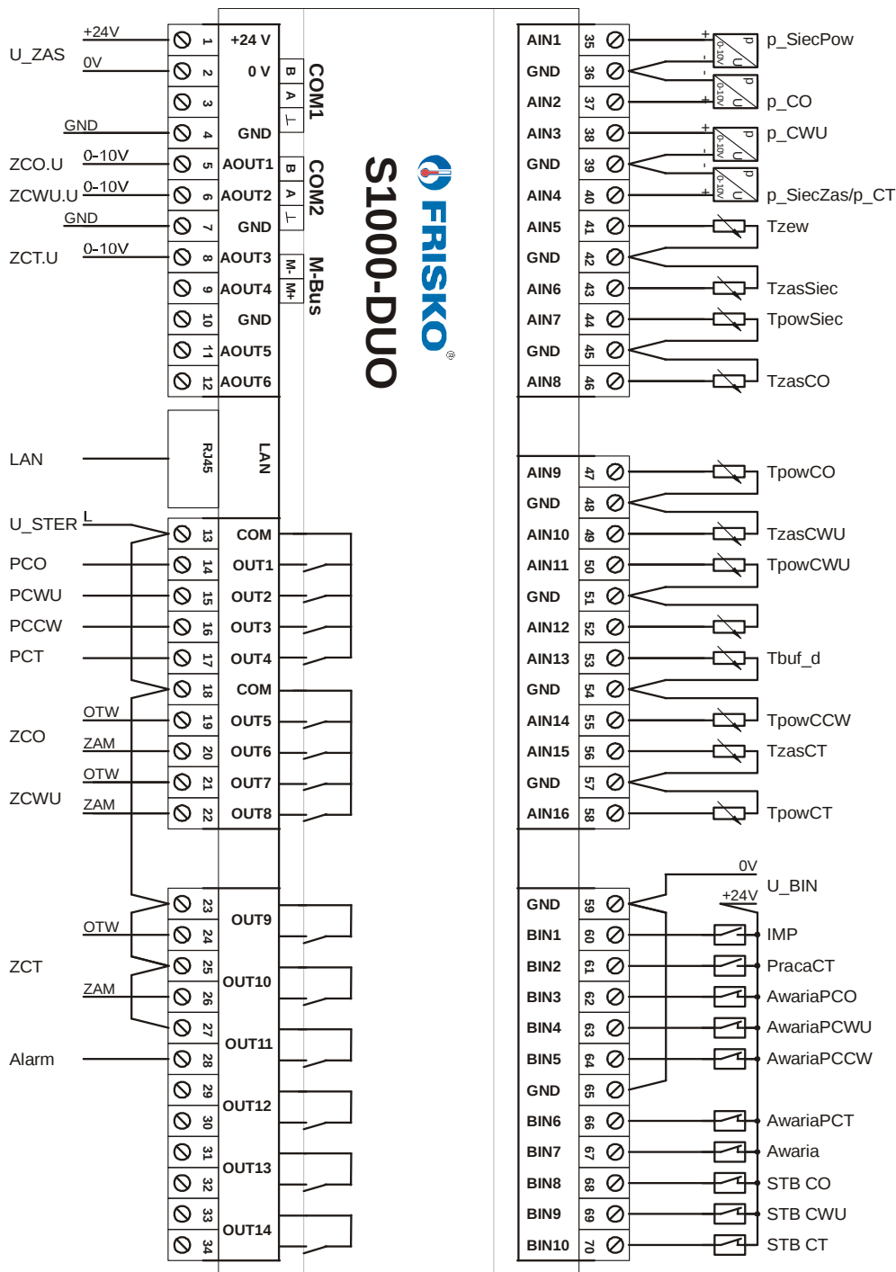
Schemat podłączeń elektrycznych regulatora S1000-DUO
